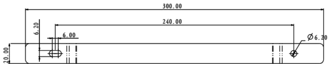
图8 臭氧仪主体安装片尺寸
