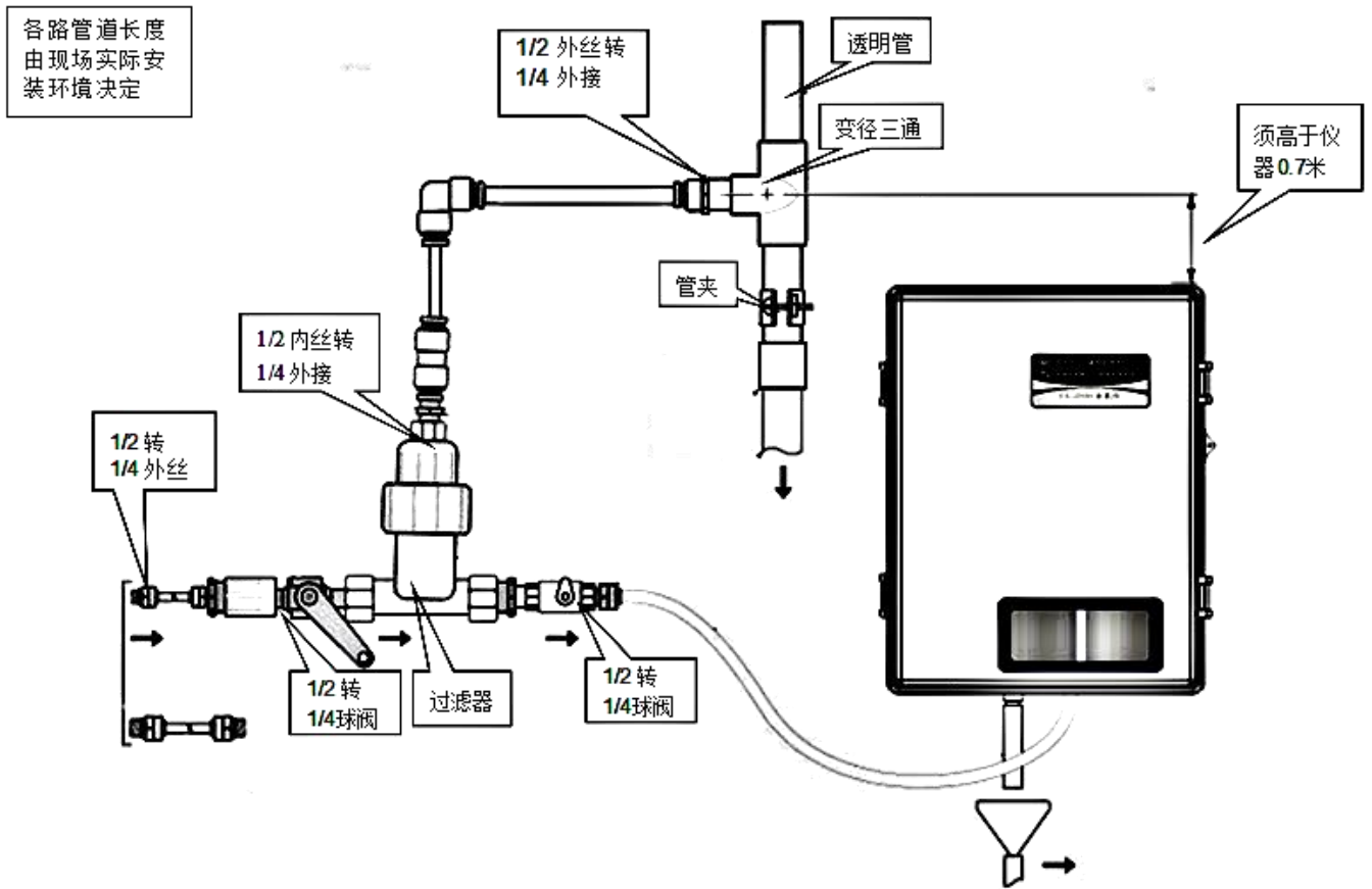
图10 臭氧仪主体水路连接示意图
